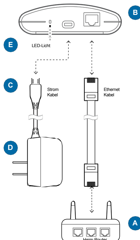
GATEWAY ULTRA Modul (Seitenansicht)
